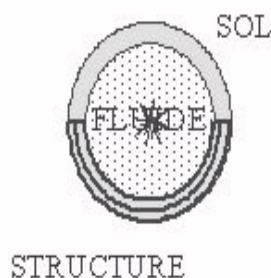
Figure 1.1-a : Domaine de la boule de dimensions finies remplie de fluide
