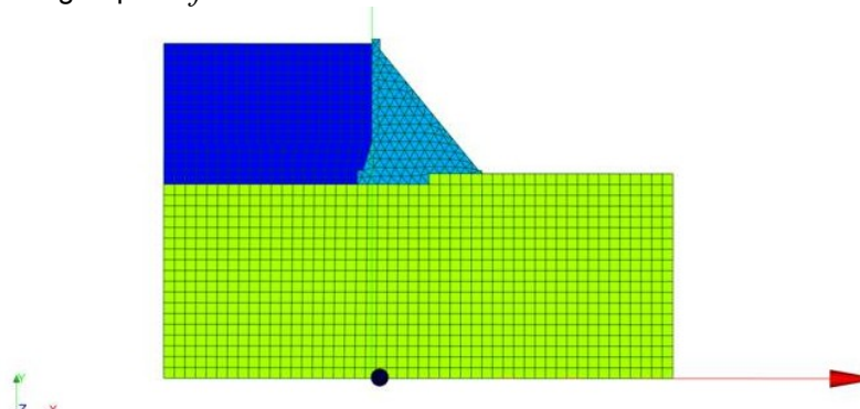
Figure 13.1-a : modèle complet 2D « full-FEM » du barrage, du sol et de sa retenue
