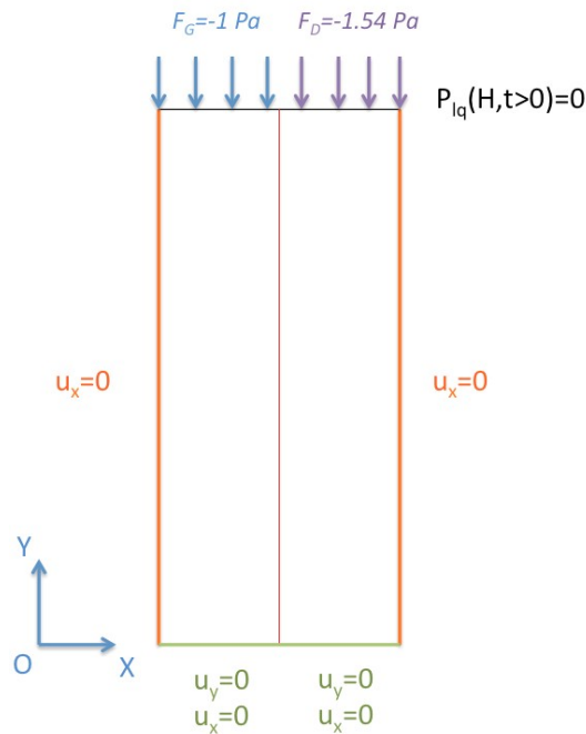
Figure 1.4.3-1 Conditions aux limites et initiales pour la modélisation 2D
