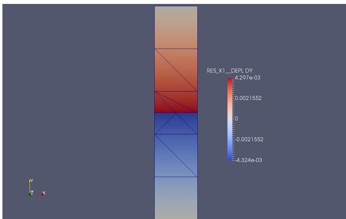
Figure 3.3-a: Champ de déplacements selon la direction (Oy)
