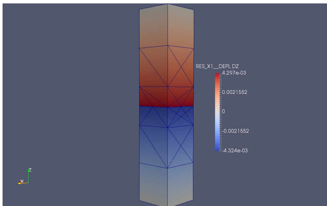
Figure 5.3-a: Champ de déplacements selon la direction (Oz)
