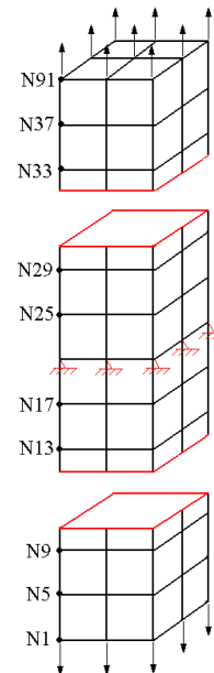
Figure 2.4-1: Maillage final et positionnement des nœuds testés
