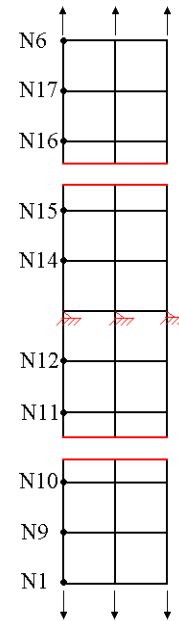
Figure 5.4-1: Maillage final et positionnement des nœuds testés
