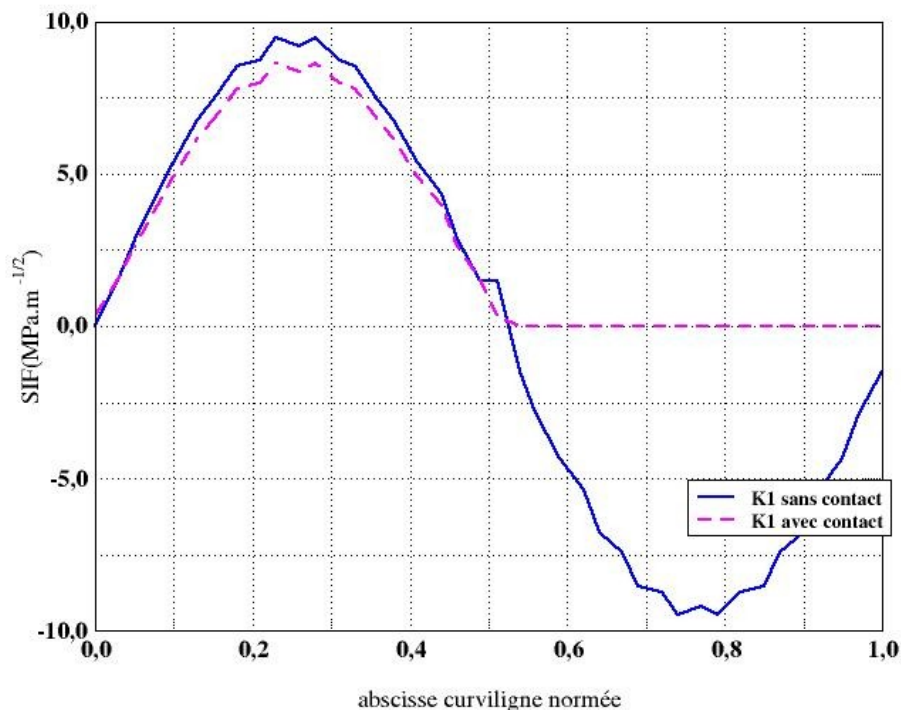
Figure 4.2 - b : K1 le long du fond de fissure (en \text{MPa.m}^{1/2} )
