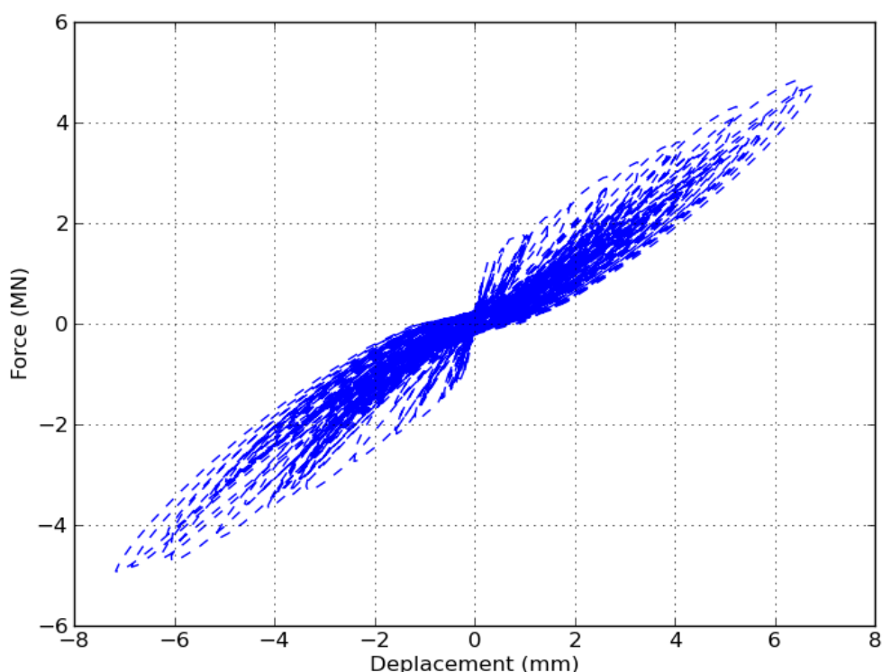
Figure 2.1-1: Réponse expérimentale du voile SAFE T5.
