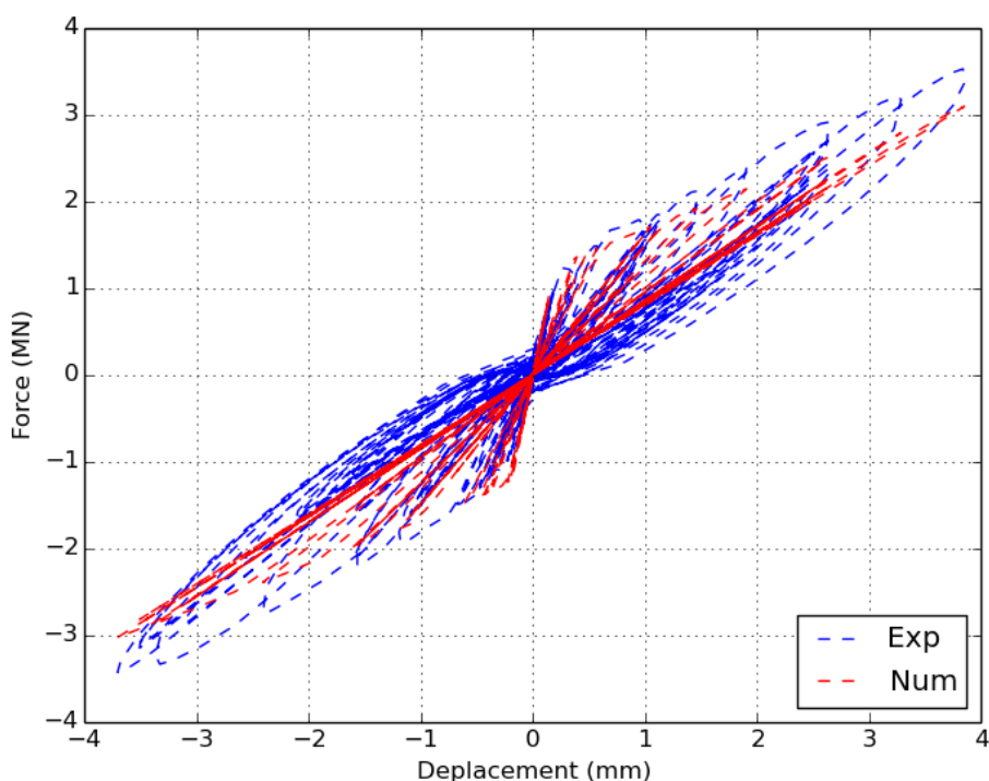
Figure 4.4-1: Comparaison de la réponse du modèle DHRC avec les données expérimentales
