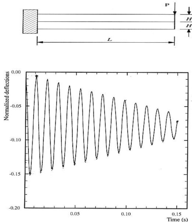
Figure : Solution en déplacement vertical du calcul de référence (Extrait de [1]).
