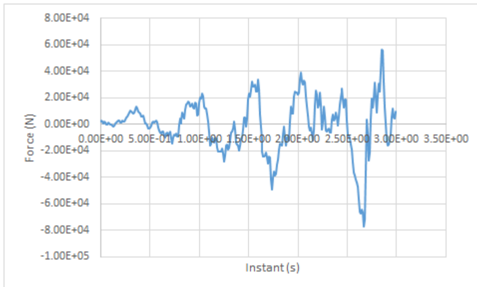
Figure 4.2-a : réaction d'appui en A en fonction du temps pour les trois premières secondes.
