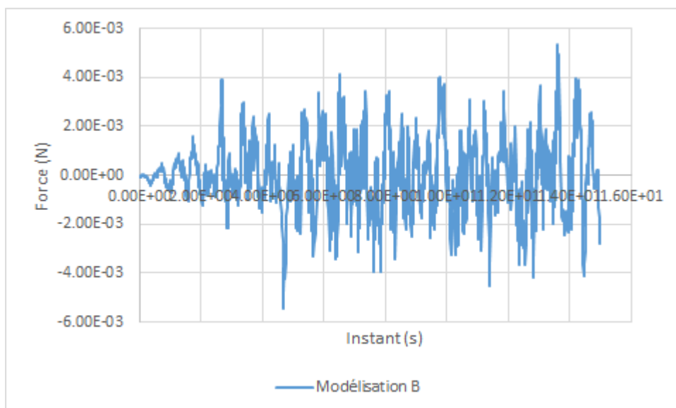
Figure 4.2-e : f lèche au centre en fonction du temps, pour 15 secondes.
