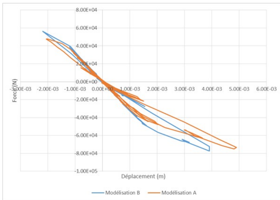
Figure 5-a: courbe réaction-flèche pour trois secondes.
