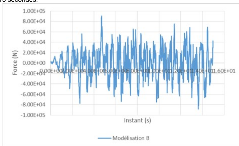
Figure 4.2-d : réaction d'appui en A en fonction du temps, pour 15 secondes.
