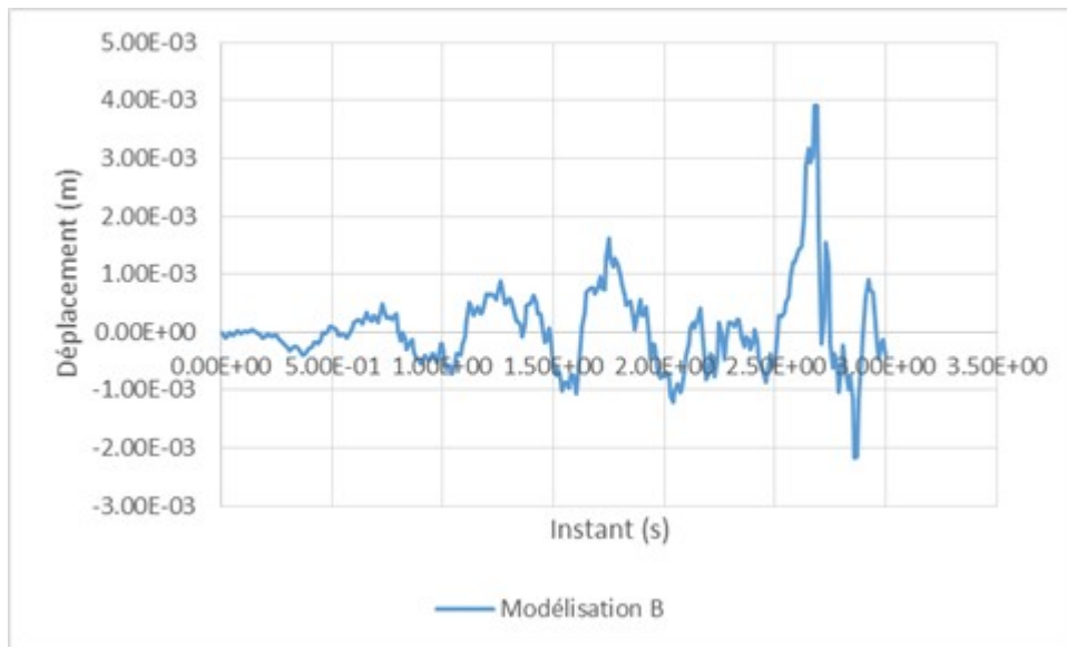
Figure 4.2-b : flèche au centre en fonction du temps pour les trois premières secondes.
