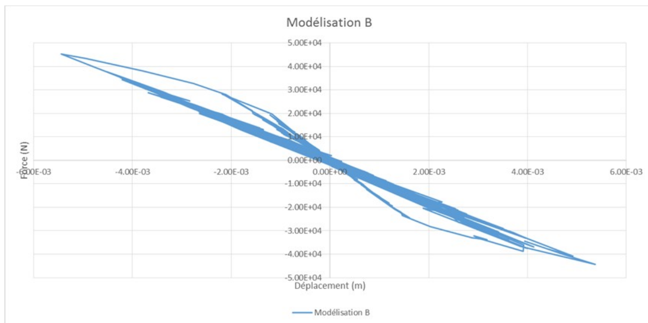
Figure 4.2-f : courbe réaction-flèche, pour 15 secondes.
