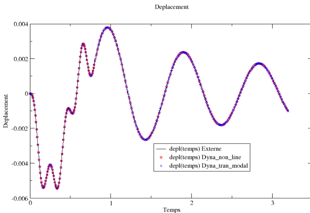
Figure 4.2-a : Réponses (déplacement en fonction du temps) calculées par une méthode externe et par Code_Aster avec les commandes DYNA_NON_LINE et DYNA_VIBRA .
