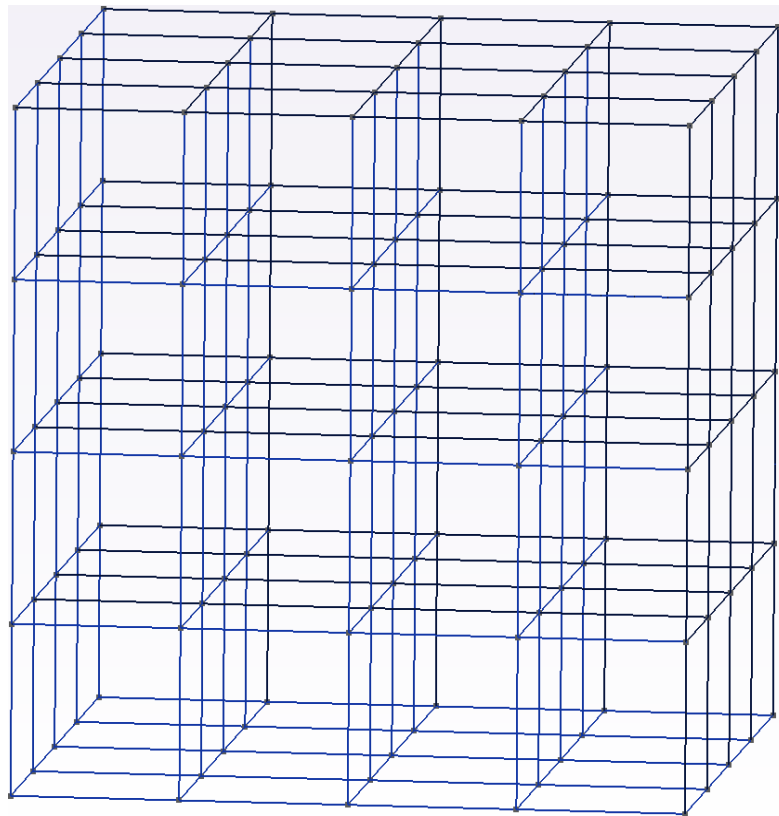
Figure 3.2-1: maillage linéaire
