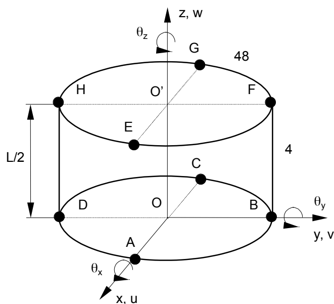
Modélisation COQUE_3D (QUAD9)
