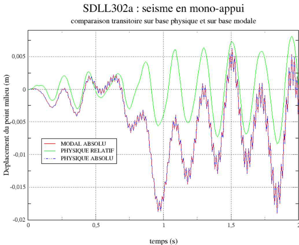
Illustration 2: SDLL302a : comparaison transitoire sur base physique vs base modale
