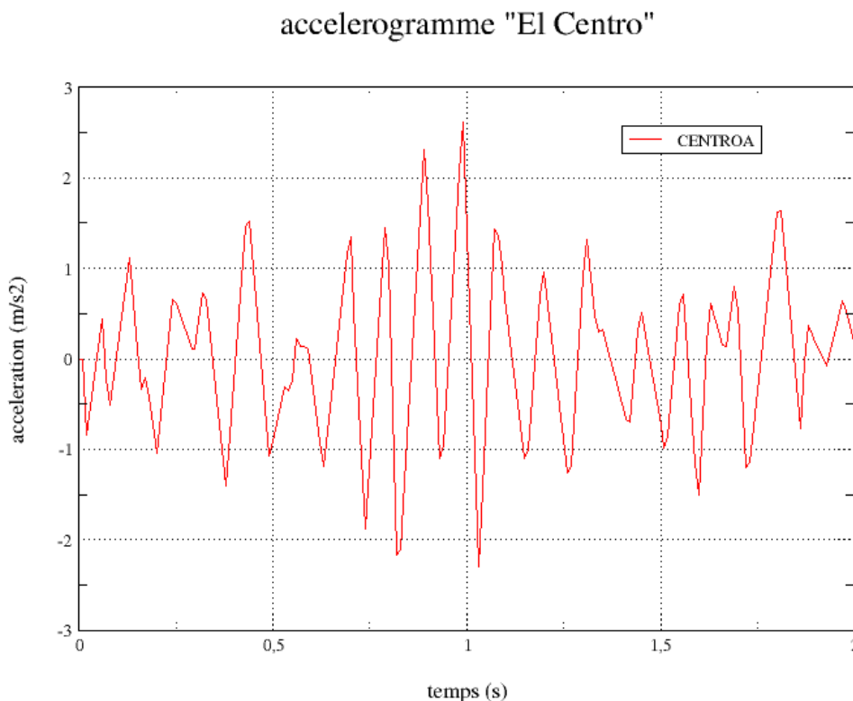
Illustration 1: Accélérogramme dit de "El Centro"
