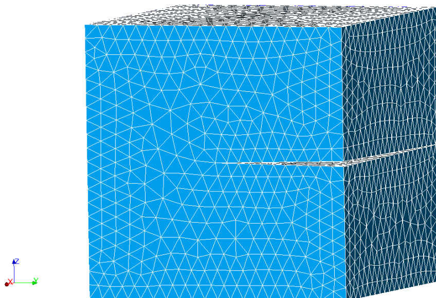
Figure 2.1-a : Maillage fissuré
