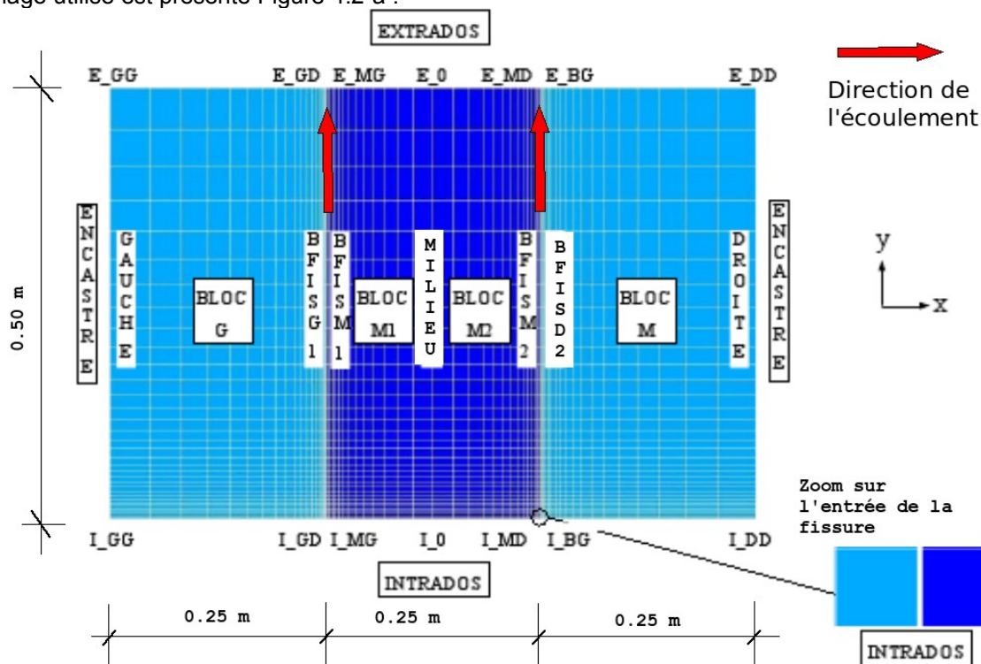
Figure 4.2-a : Maillage complet
