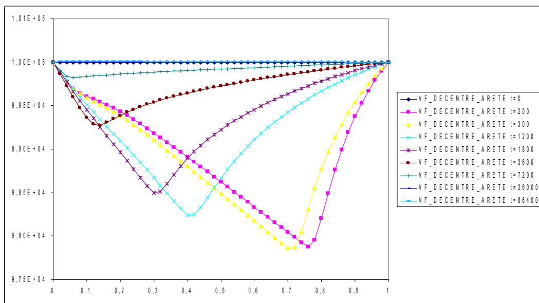
Illustration 2: Pression de gaz le long de la colonne
