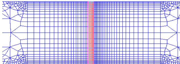
Figure 4.1-b : Maillage grossi de la jonction 16MND5-304L et détail de l'interface et de la zone décarburée
