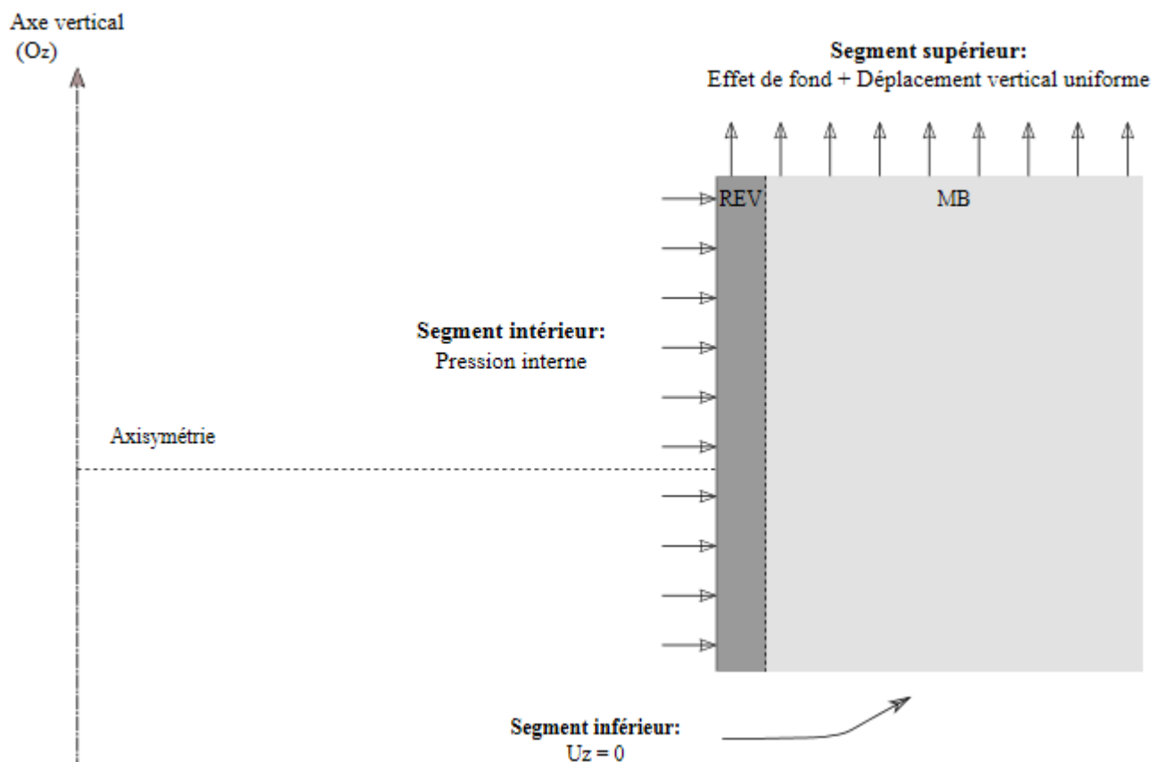
Figure 1.3-b: Problème mécanique considéré
