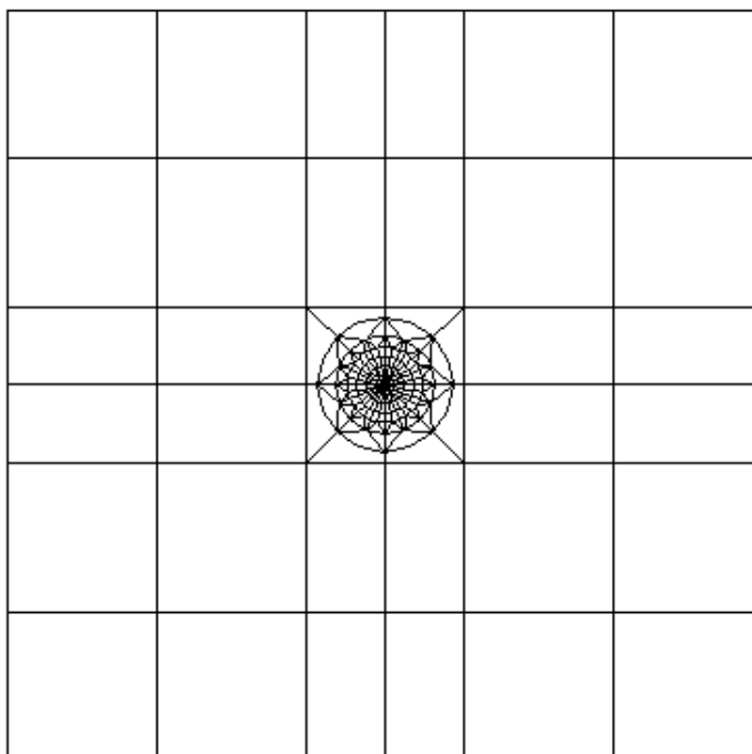
Maillage complet - Modélisation E
