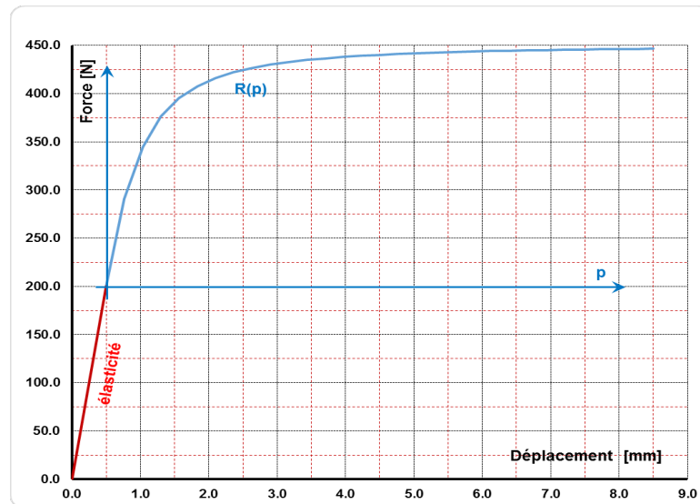
Figure 1.3.1-a : Comportement non-linéaire
