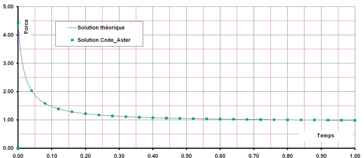
Figure 5.5-a : Courbes de fluage théorique et calculée par Code_Aster.
