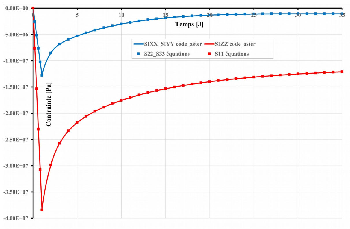
Figure 5.2-a : Compression sur cube confiné, comparaison entre code_aster et la solution théorique.
