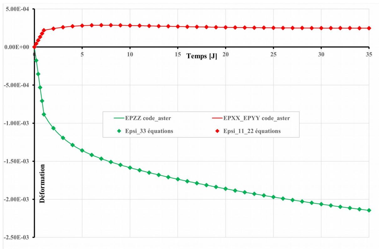
Figure 2.2-a : Compression sur cube libre, comparaison entre code_aster et la solution théorique.
