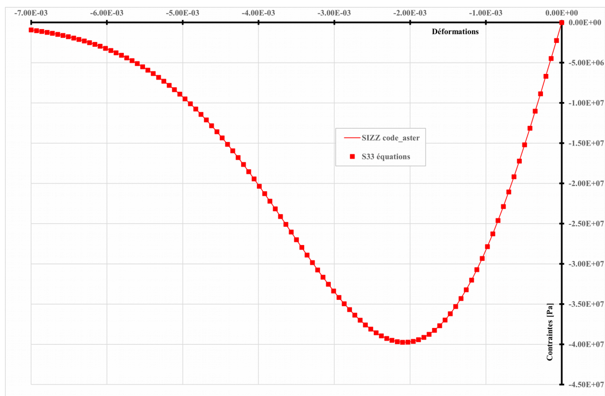
Figure 3.2-a : Compression sur cube libre, comparaison entre code_aster et la solution théorique.
