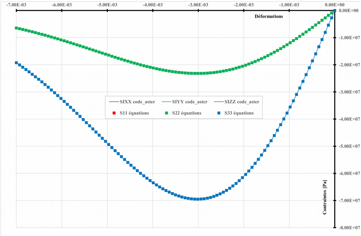
5.2-a : Compression sur cube confiné, comparaison entre code_aster et la solution théorique.
