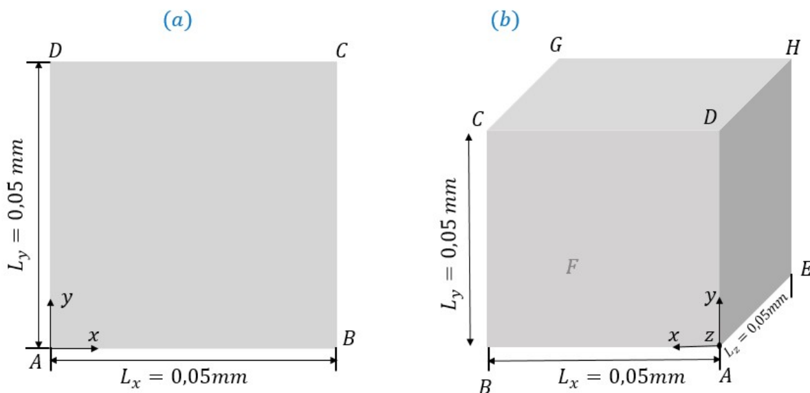
Figure 1.1-a: Géométries d'un carré (a) et d'un cube (b)
