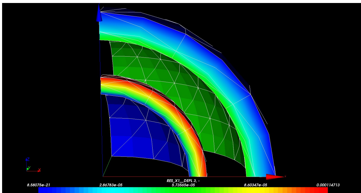
Figure 4.3-a : Champ de déplacement radial
