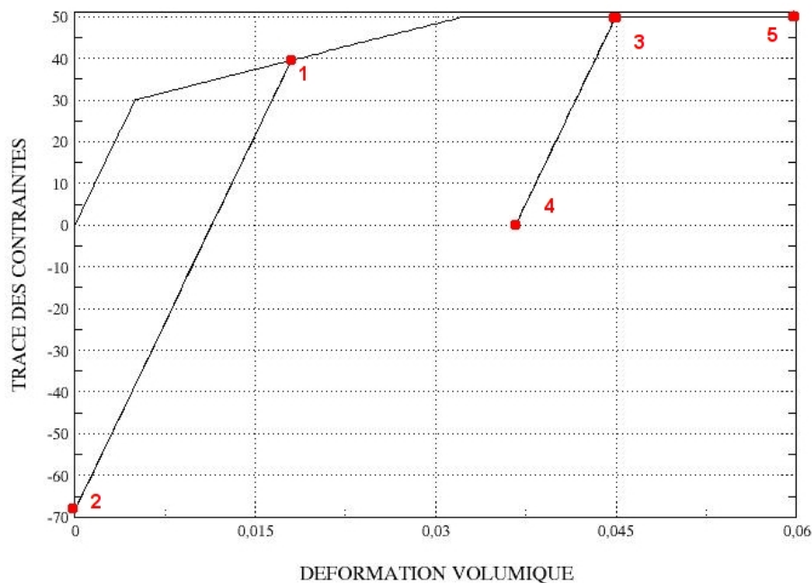
Figure 2.2.5-a: courbes contrainte-déformation pour écouissage linéaire.
