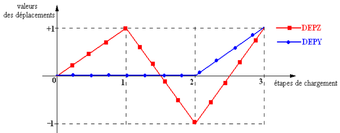
Figure 1.3-1: Variations des chargements en déplacements imposés
