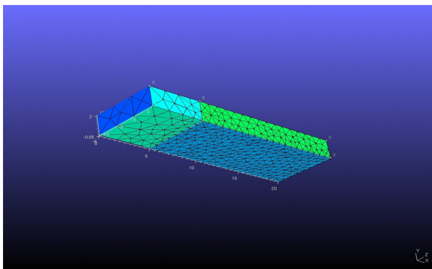
Figure 5.2-a : Schéma du maillage de la demi poutre, (la fissure initiale n'est pas maillée).
