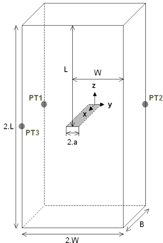
Figure 1.1-1 : Eprouvette avec fissure centrale débouchante
