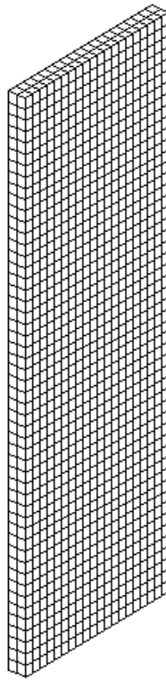
Figure 11.1-a : Maillage 2 \times 20 \times 51 HEXA8
