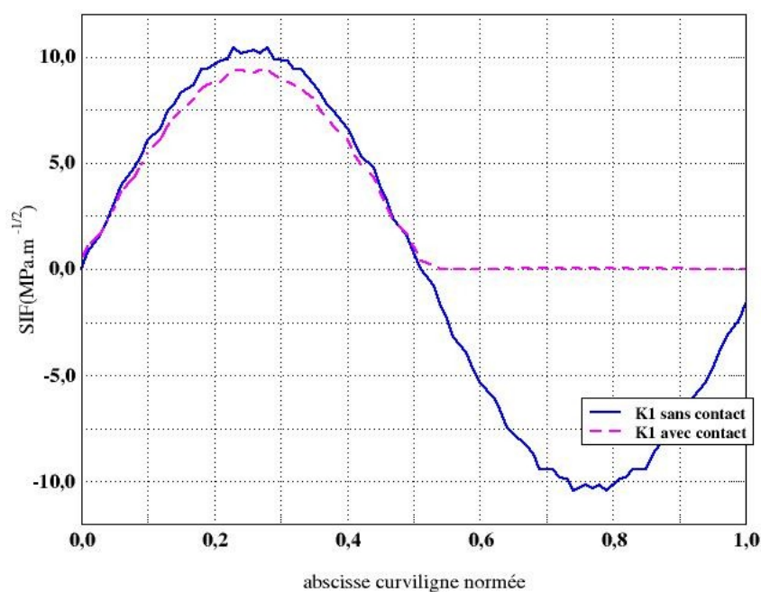
Figure 4.4-b : K1 le long du fond de fissure (en \text{MPa.m}^{1/2} )
