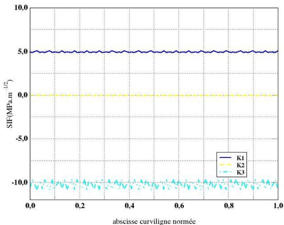
Figure 4.4-a : K1 , K2 et K3 le long du fond de fissure (en \text{MPa.m}^{1/2} )
