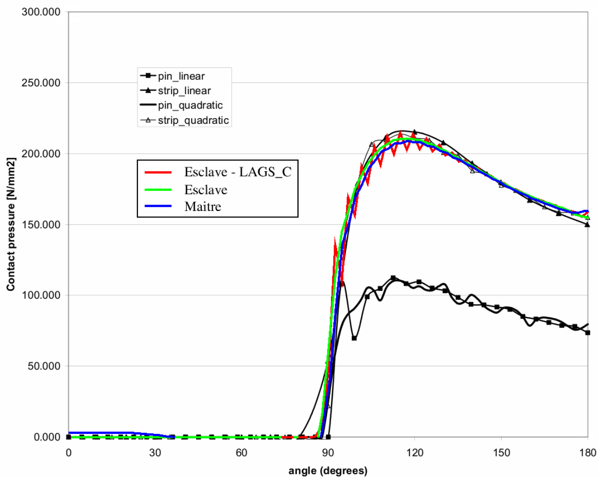
Illustration 3: comparaison entre MARC et Code_Aster (pression de contact sur le poinçon)
