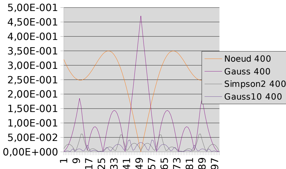
Figure 9.3-1: Évolution de la pression de contact lors de la rotation pour 1600 éléments sur la circonférence R=R_2 . Une intégration avec 3 points de Gauss conduit à une erreur maximale de 45%. Une intégration nodale ne donne pas des résultats corrects lorsque les maillages maître et esclave sont compatibles. Seules les intégrations de Gauss à l'ordre 10 et de Simpson à l'ordre 4 permettent de ramener l'erreur maximale aux alentours de 5% pour des maillages incompatibles.
