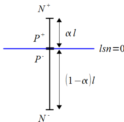
Figure 1.4.1-1: Arête intersectée par une interface
