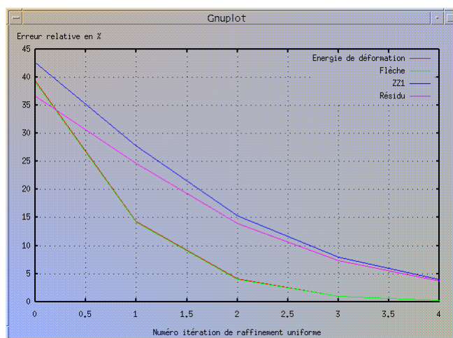
Figure 3.1-b : D  croissances des erreurs relatives de l'  nergie de d  formation et de la fl  che compar  es    celles de la composante totale relative des indicateurs.
