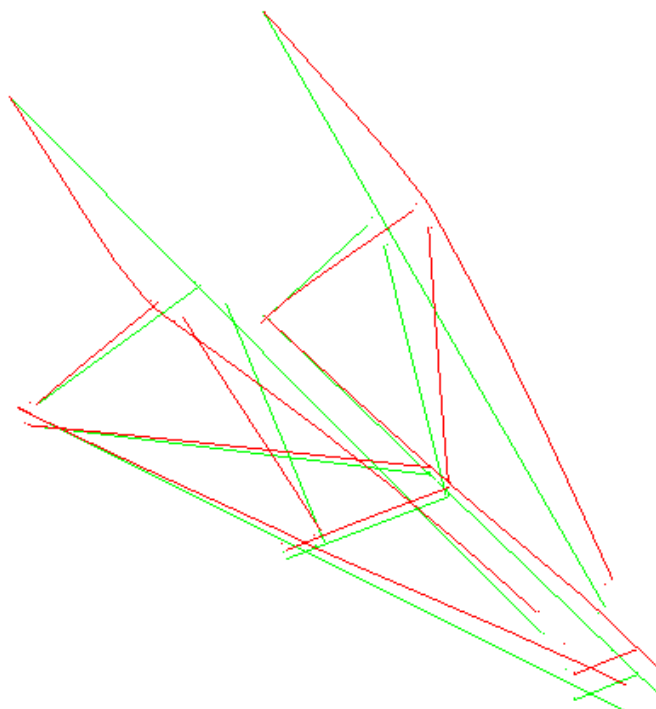
Figure 4.4.4-a : Mode de ruine prédit par le calcul en configuration C2 (amplitude 1)
