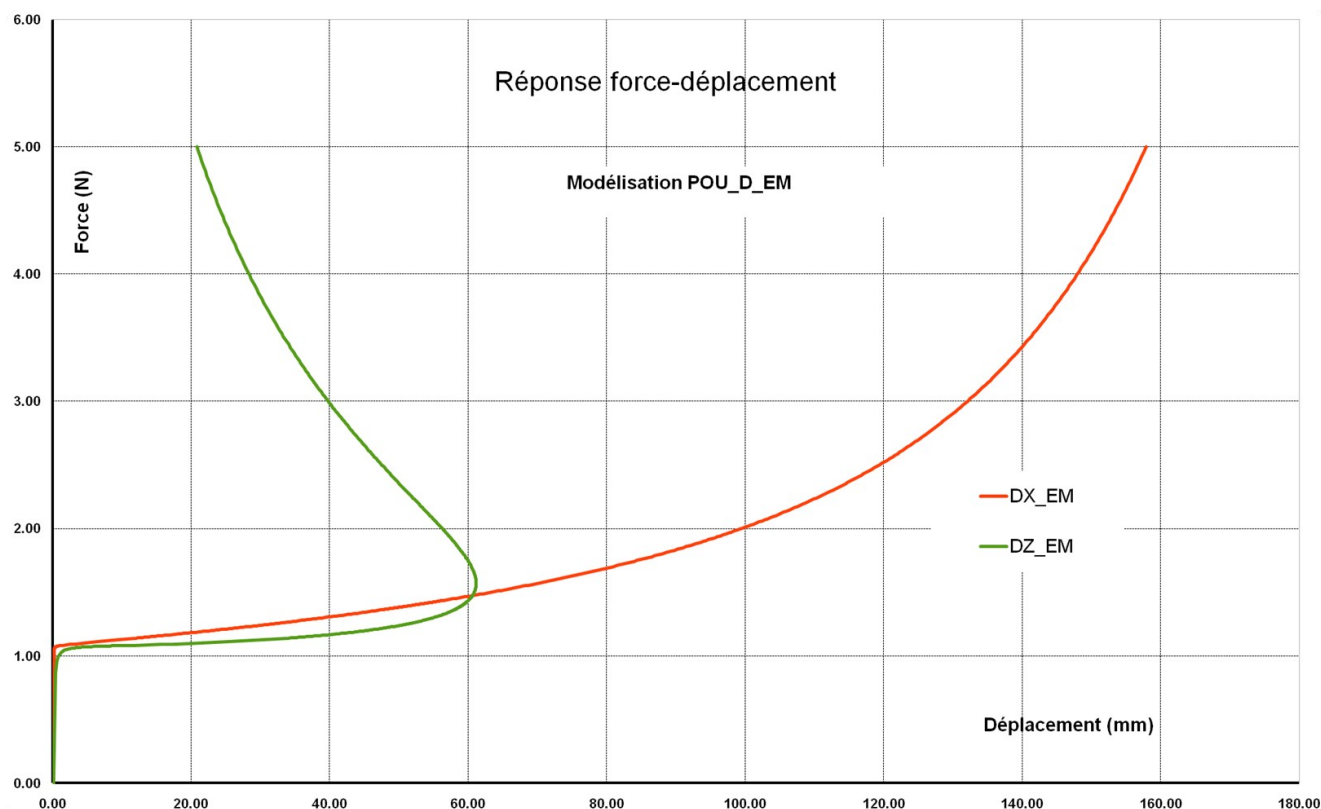
Figure 8.4.2-a : Réponse Force-Déplacement, modélisation POU_D_EM .
