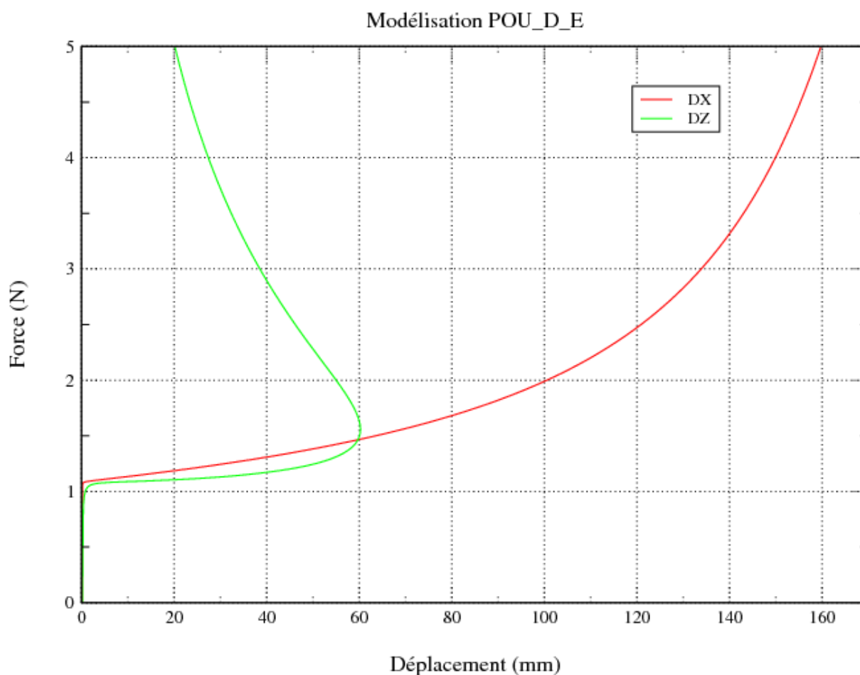
Figure 7.4.2-a : Réponse Force-Déplacement, modélisation POU_D_E.
