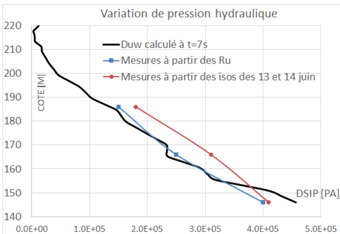
Figure 3-b : Profil de variation de pression interstitielle \Delta u_w le long d'une coupe verticale du noyau entre t = 0 et t = 7\text{sec}
