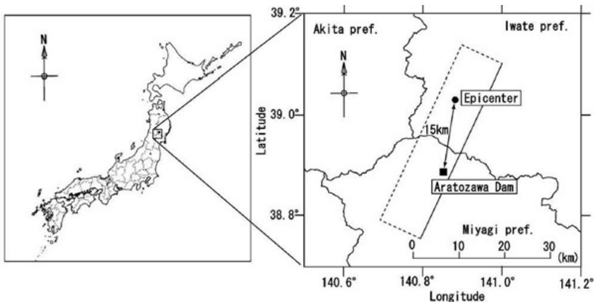
Figure 1.1.1-a : Emplacement du barrage d'Aratozawa et de l'épicentre du séisme de Miyagi, 2008 [ 3 ]
