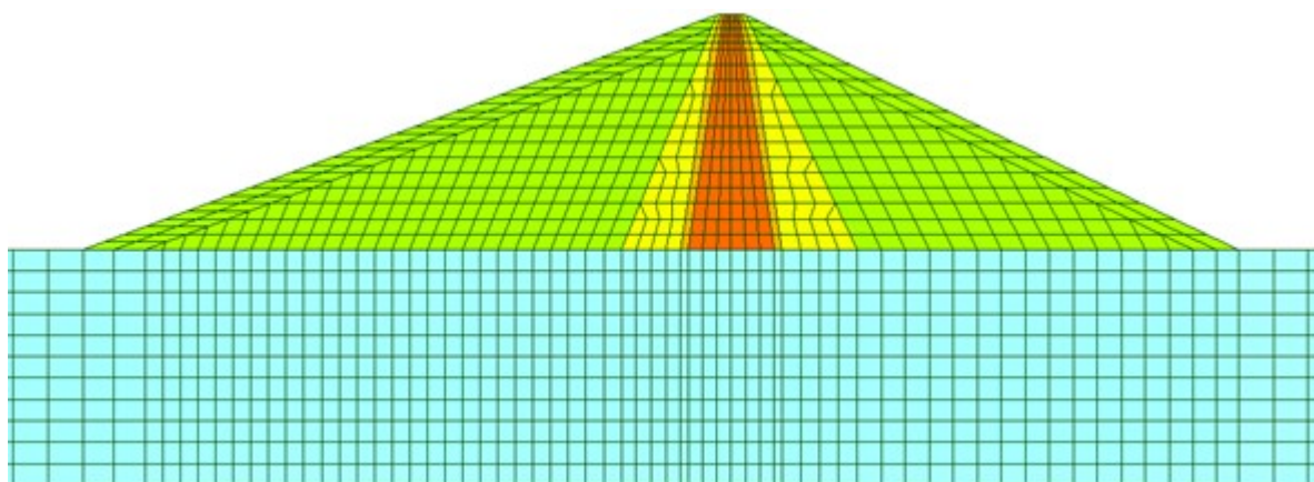
Figure 1.2-a : Maillage du barrage d'Aratozawa (en haut)
