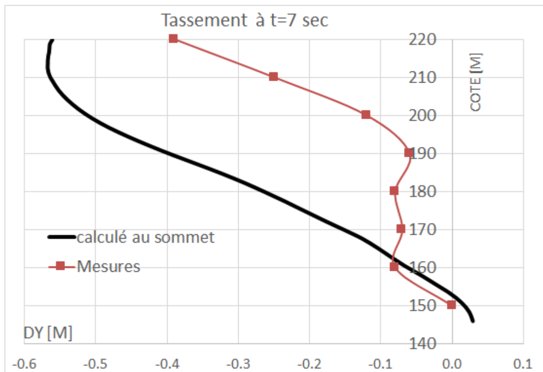
Figure 3-a : Profil de tassement \Delta u_y le long d'une coupe verticale du noyau à t = 7 sec
