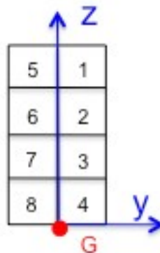
Figure 2 : Découpage de la section en 8 fibres
