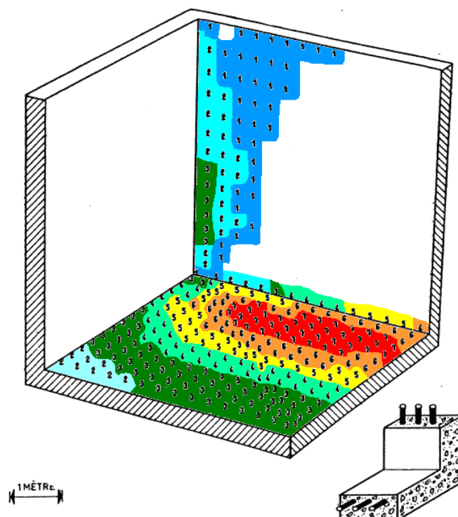
Fig. 19. — Cuve carrée en béton armé. Carte de ferrailage des aciers Y intérieurs (en \text{cm}^2 par mètre).
