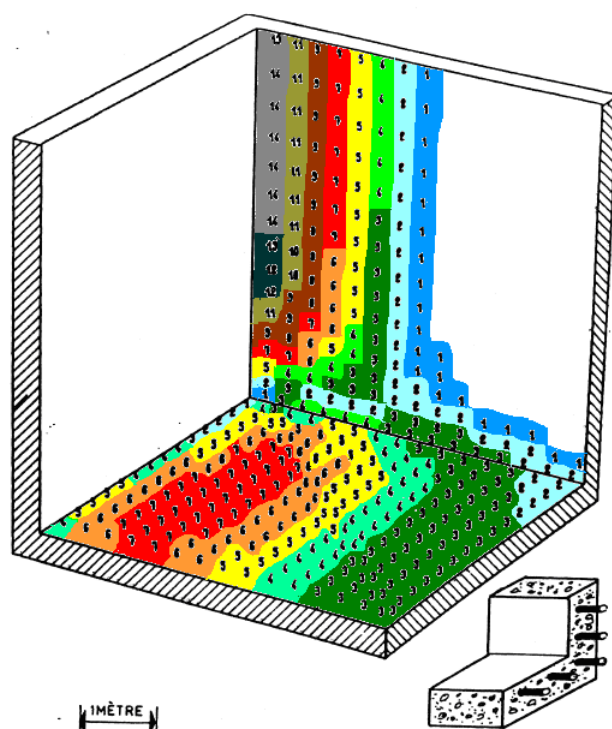
Fig. 18. — Cuve carrée en béton armé. Carte de ferrailage des aciers X intérieurs (en \text{cm}^2 par mètre).
