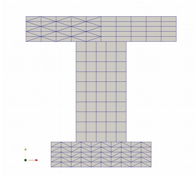
Figure 4-1: Section de la poutre pour SSL111b
