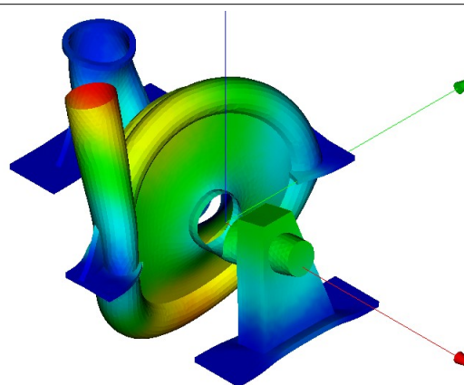
Illustration 12: Mode 2 du calcul SSD par la méthode des interfaces
