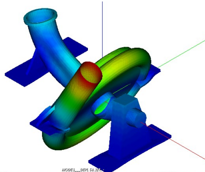
Illustration 4: Mode 1 du calcul SSD par Craig et Bampton
