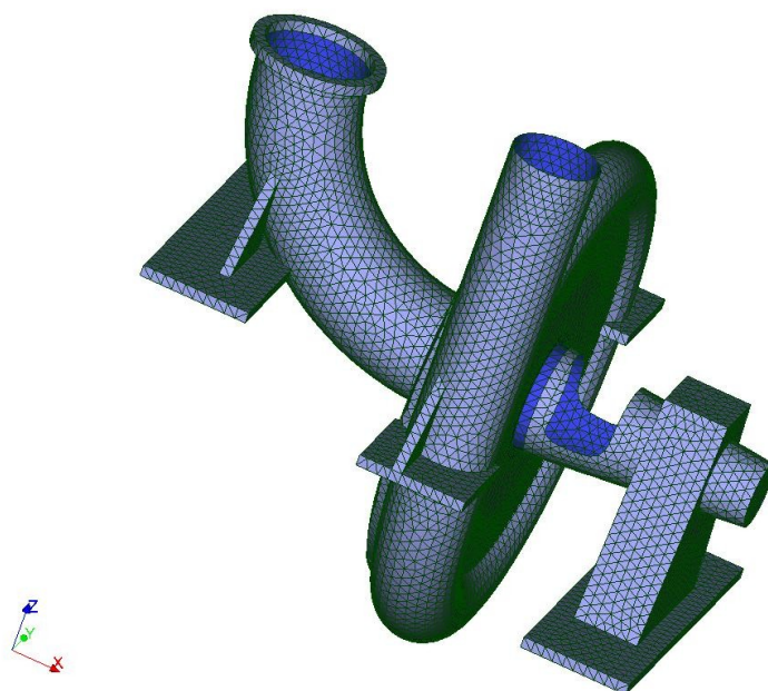
Illustration 2: Pompe complète
