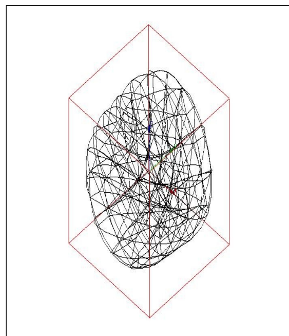
Déformée modale ( 2469.64 Hz )
