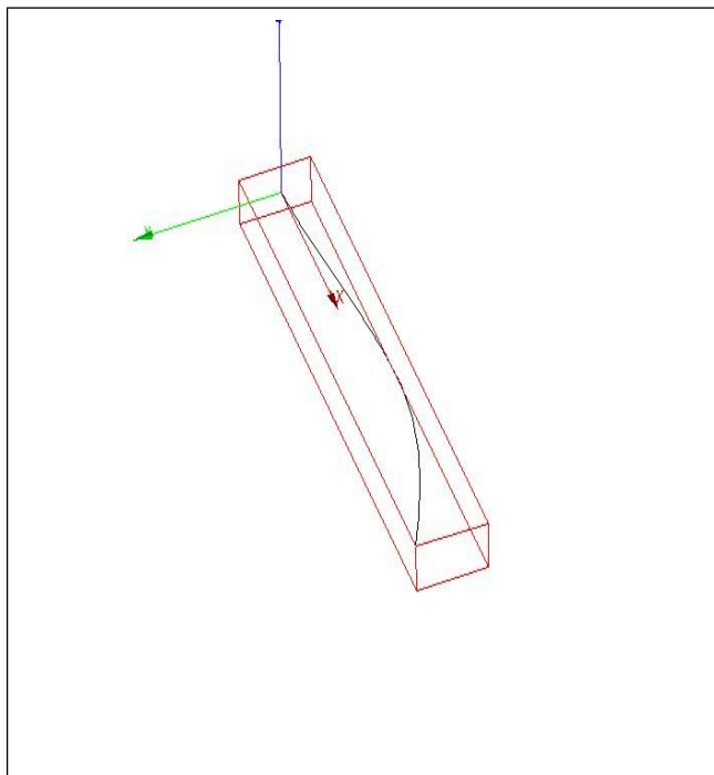
Déformée modale ( 1050.60 Hz )
