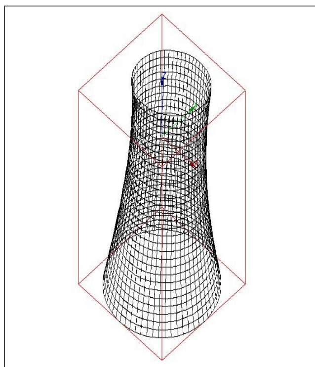
Déformée modale ( 2.80065 Hz )
