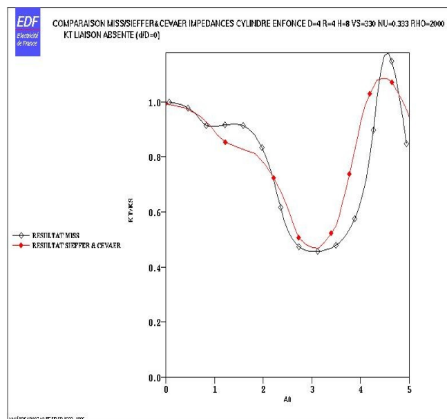
Figure 4.1-d : Évolutions des impédances de torsion
