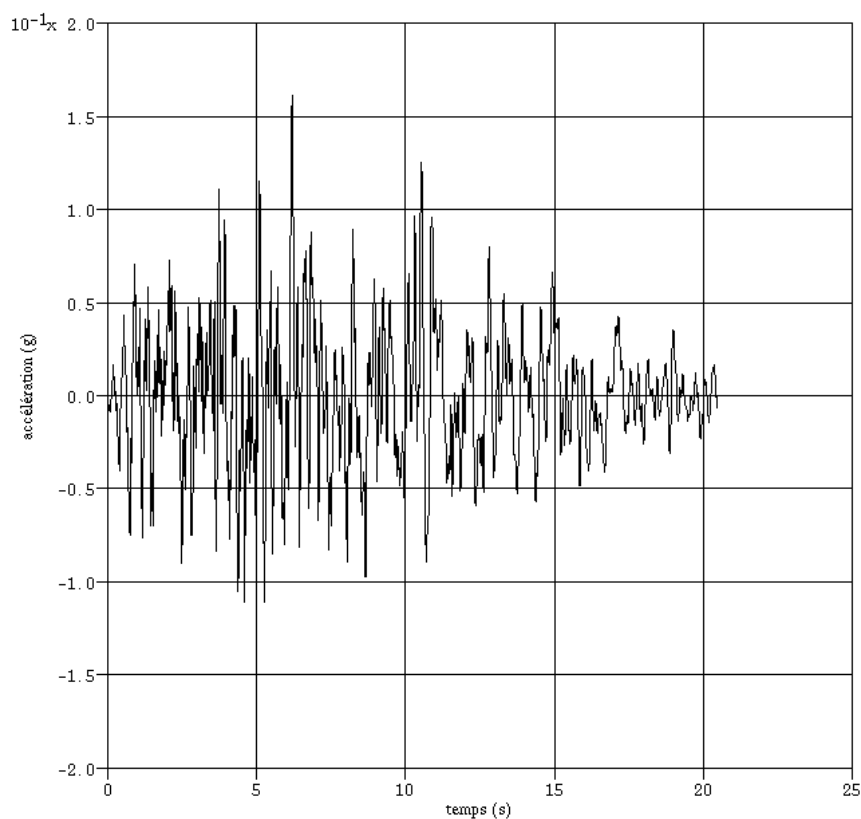
Figure 1.3-c : Accélérogramme acc3.c2
