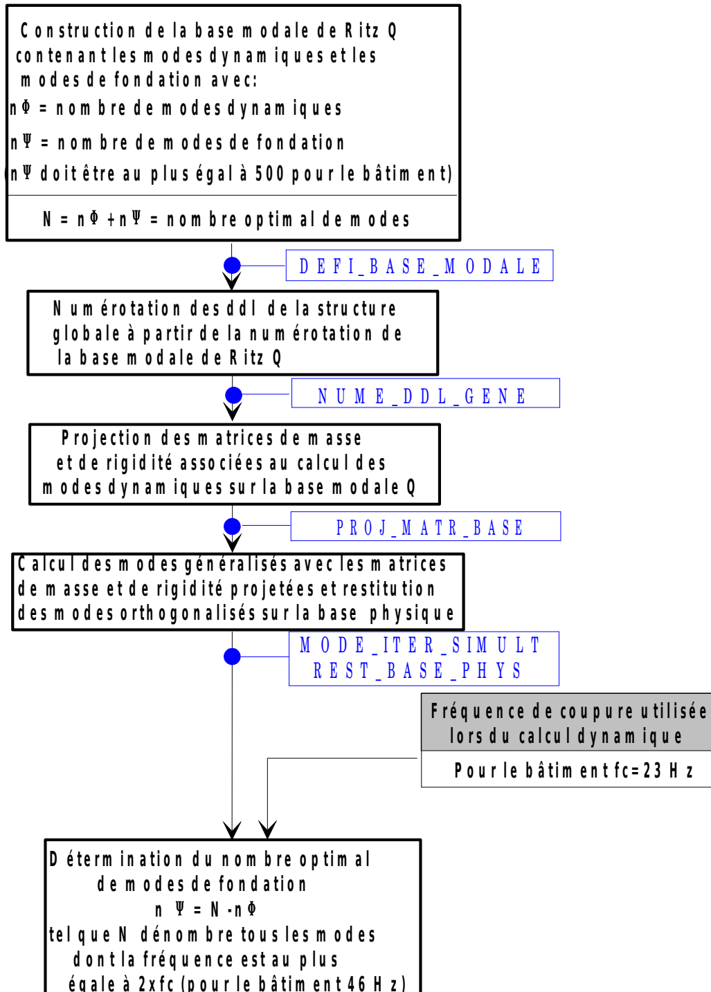
Figure 2.1.5-a : Optimisation du nombre de modes de fondation
