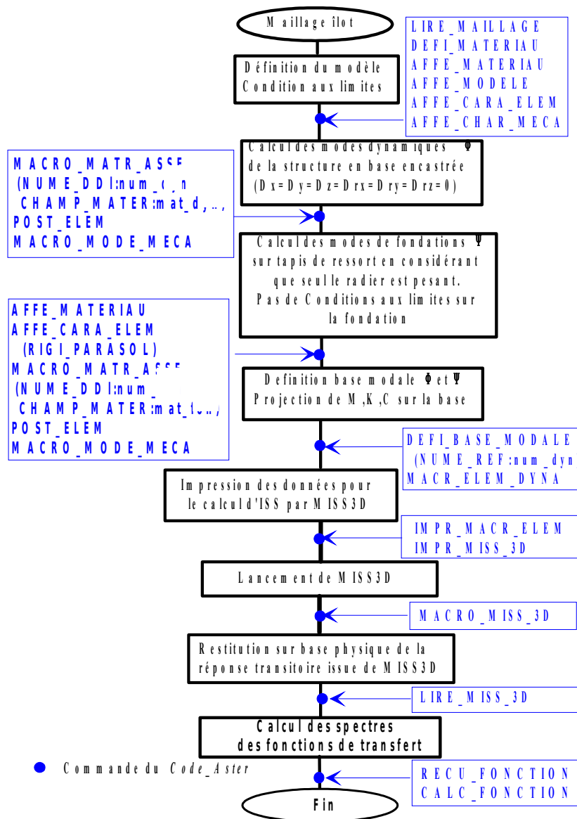
Figure 2.1.5-b : Synoptique du calcul avec modes de fondation sur tapis de ressorts
