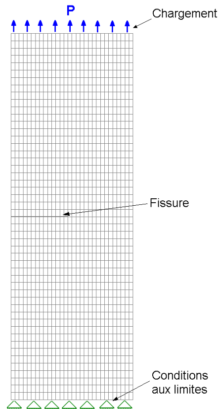
Figure 3.2-a: Maillage pour la modélisation A. Illustration des conditions aux limites et du chargement
