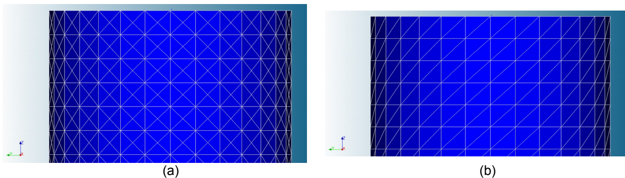
Fig. 5. Exemples des maillages en triangle
