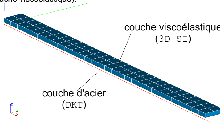
Image 3.1-1 : Maillage de la structure.
