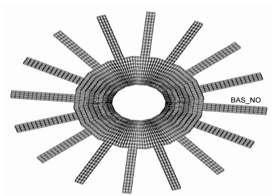
Figure 3.1. Maillage de la modélisation A
