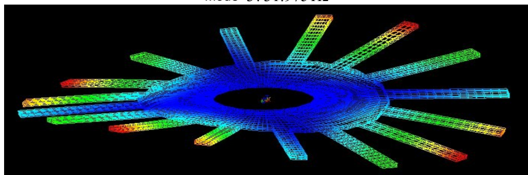
Mode 4 : 33.4833 Hz
