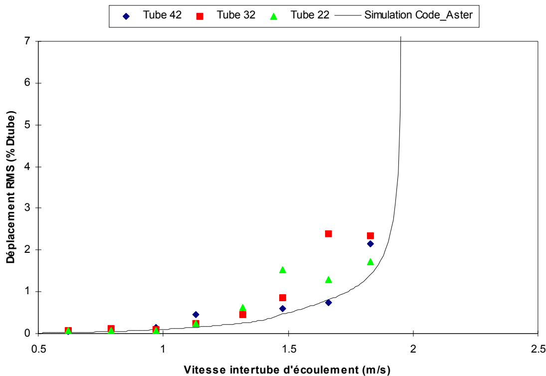
Figure 5.1-a : Déplacement RMS au point E, en fonction de la vitesse intertube d'écoulement, exprimé en pourcentage du diamètre extérieur du tube.
